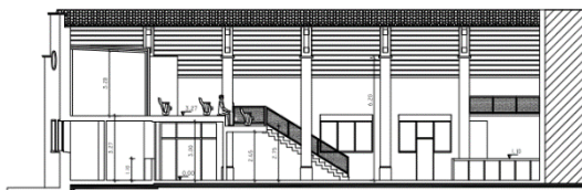
SEZIONE A - A
