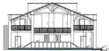
SEZIONE D - D
