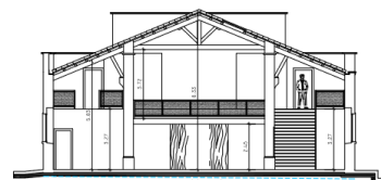
SEZIONE D - D
